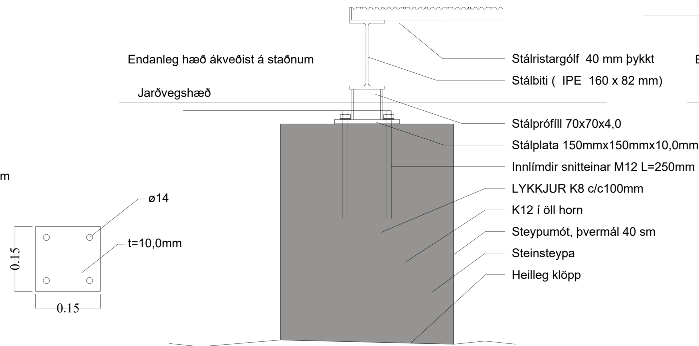
SNIÐ Í STEYPTA UNDIRSTÖÐU MKV.1:5
