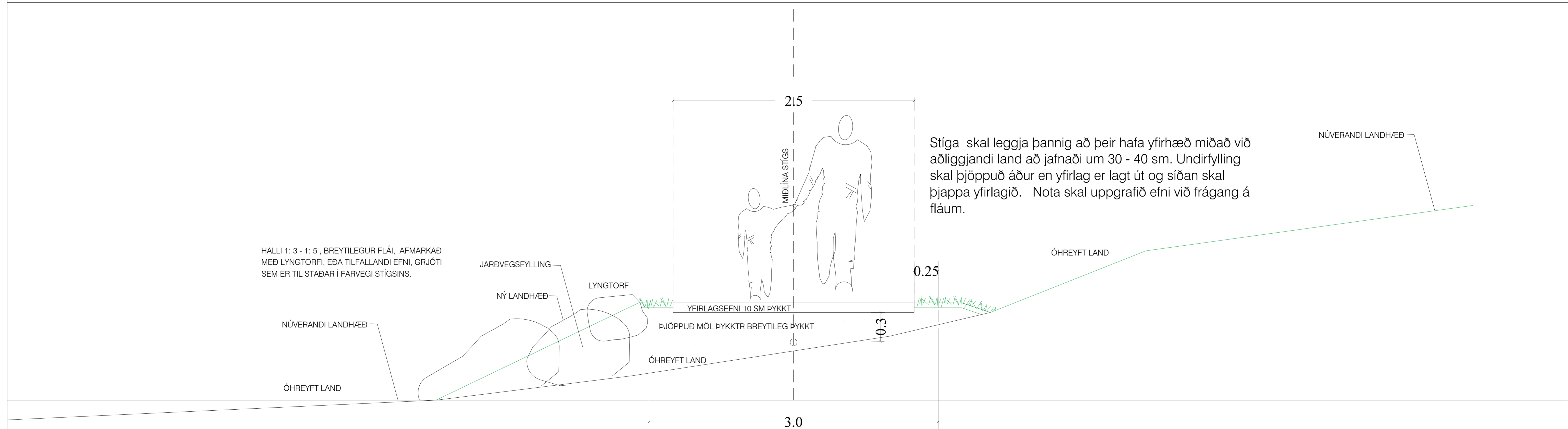
Stígar - Prinsippið sýnir stíg sem er 2.5 metrar á breidd. Hér er sýnt prinsipp með grjóti til þess að taka upp hæðamun að svæði sem við viljum ekki raska. Mkv.1:20
