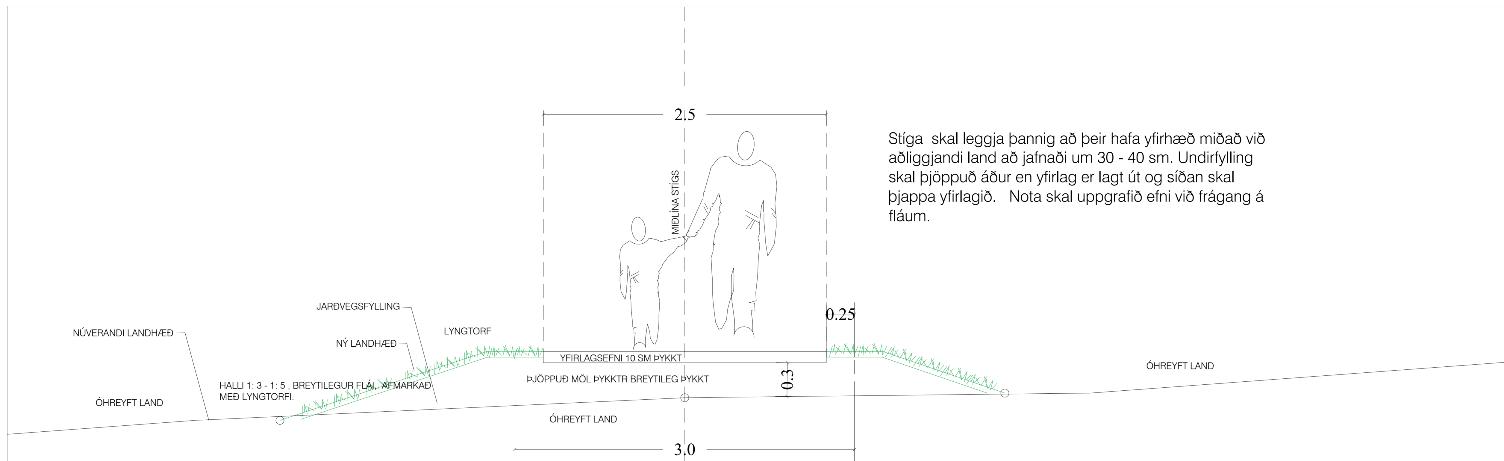
Stígar - Prinsippið sýnir stíg sem er 2.5 metrar á breidd. Mkv.1:20
