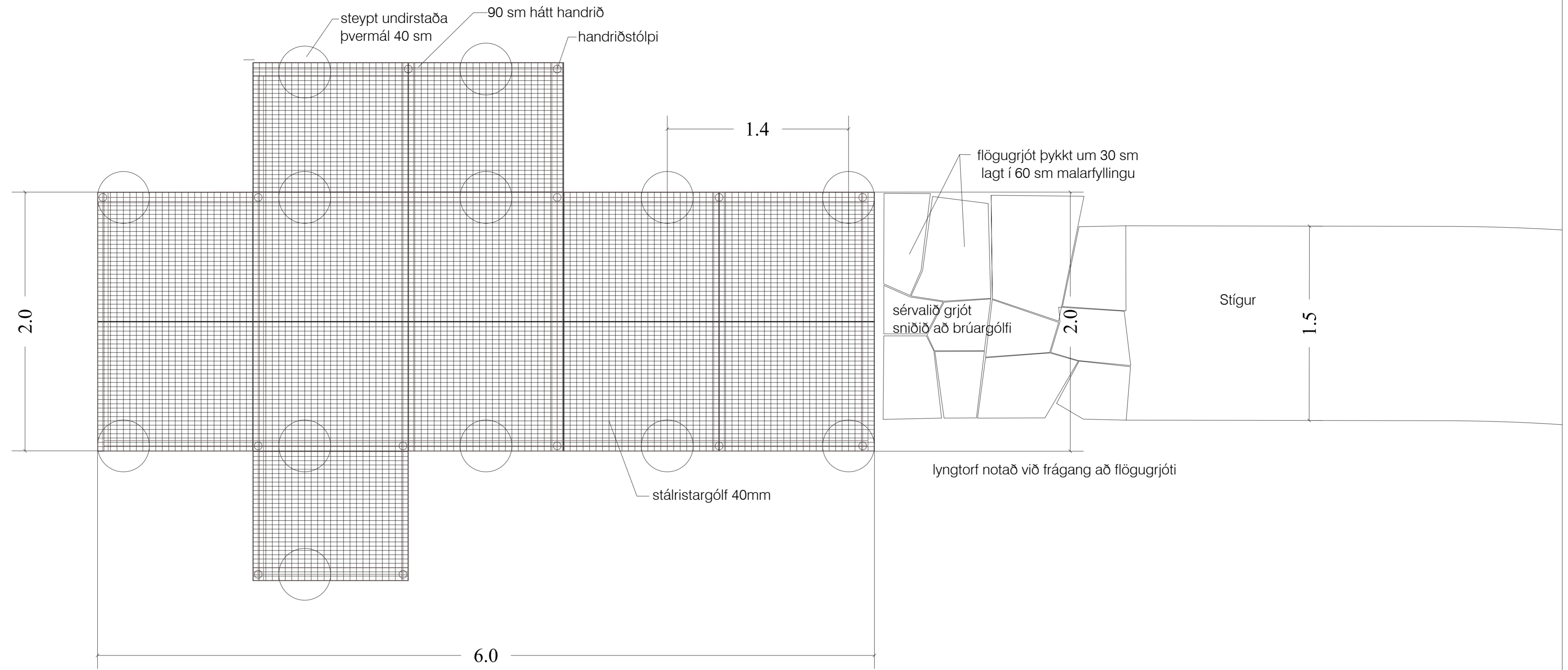
Útsýnispallur I undirbygging mkv: 1. 20
