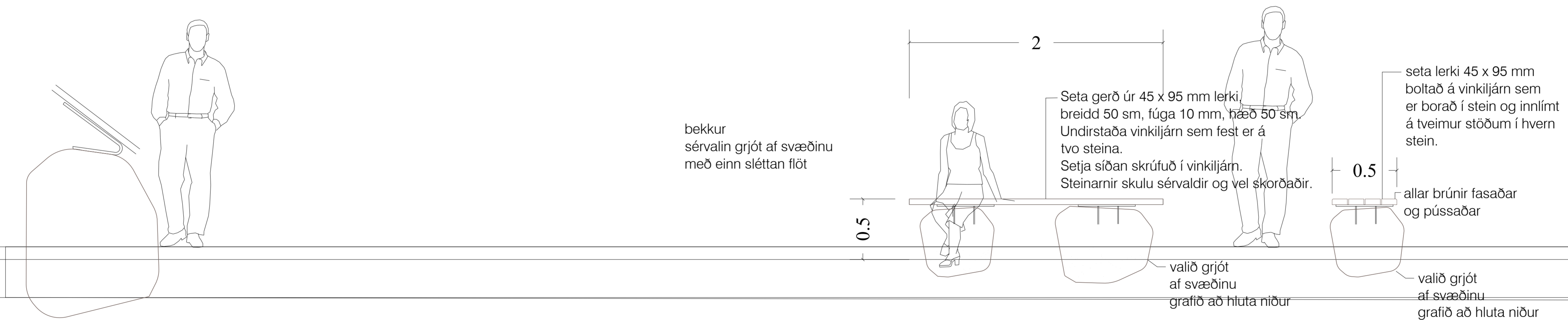
Deili í bekk mkv 1:20
