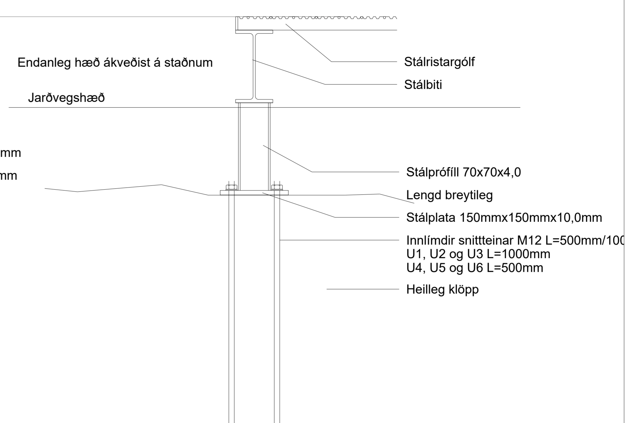
SNIÐ Í UNDIRSTÖÐU Í KLÖPP MKV.1:5
