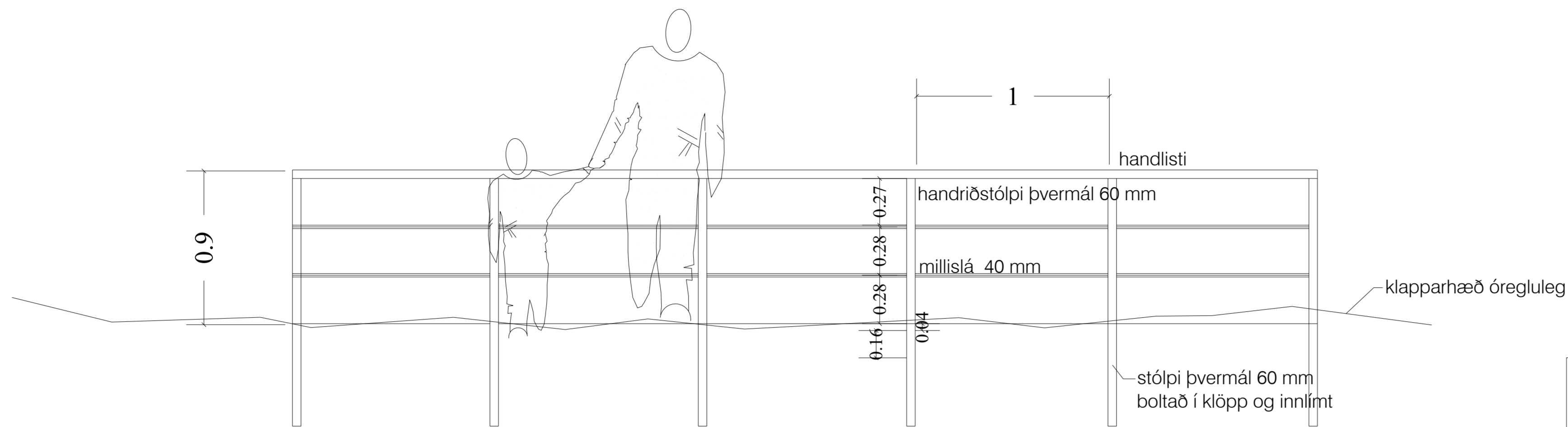
Útsýnispallur ásýnd á handlista mkv: 1. 20
