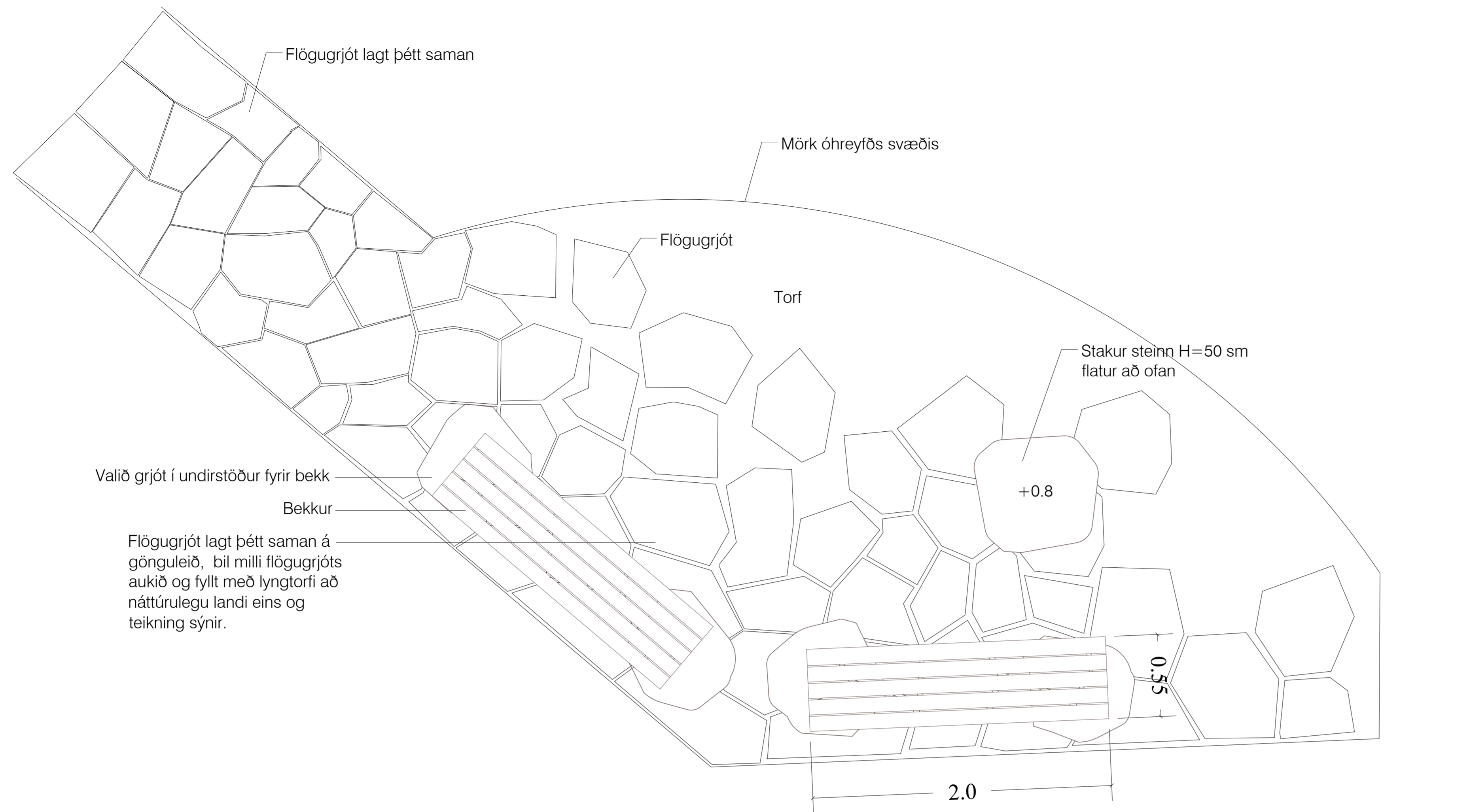
Yfirlitsmynd af áningarsvæði með bekkjum og flögugrjóti 1:20
