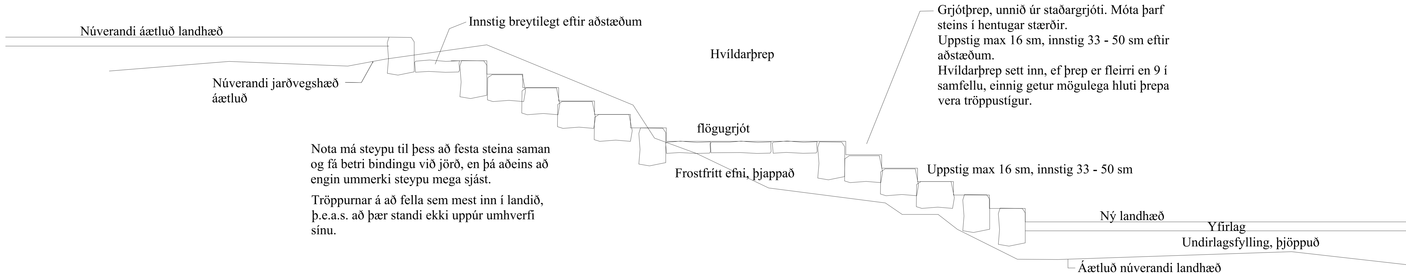
DÆMIGERT SNIÐ Í FRÁGANG Á STEINTRÖPPUM MKV.1:20
