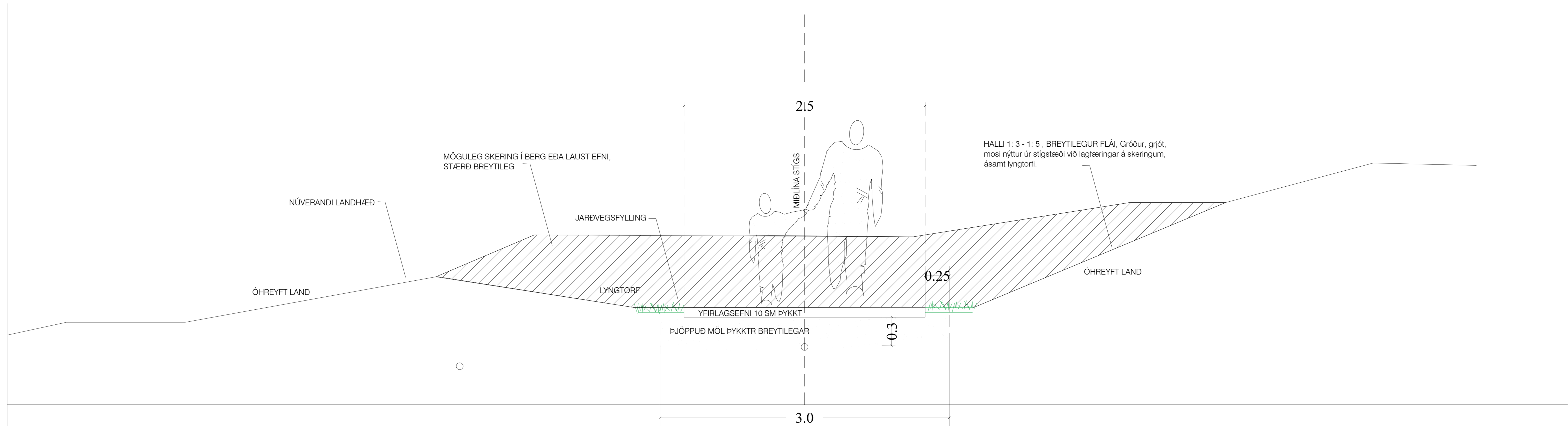
Prinsippið sýnir stíg sem er 2.5 metrar á breidd sem liggur í skeringu í landslaginu. Skravering sýnir mögulegt úrtak. Mkv.1:20
