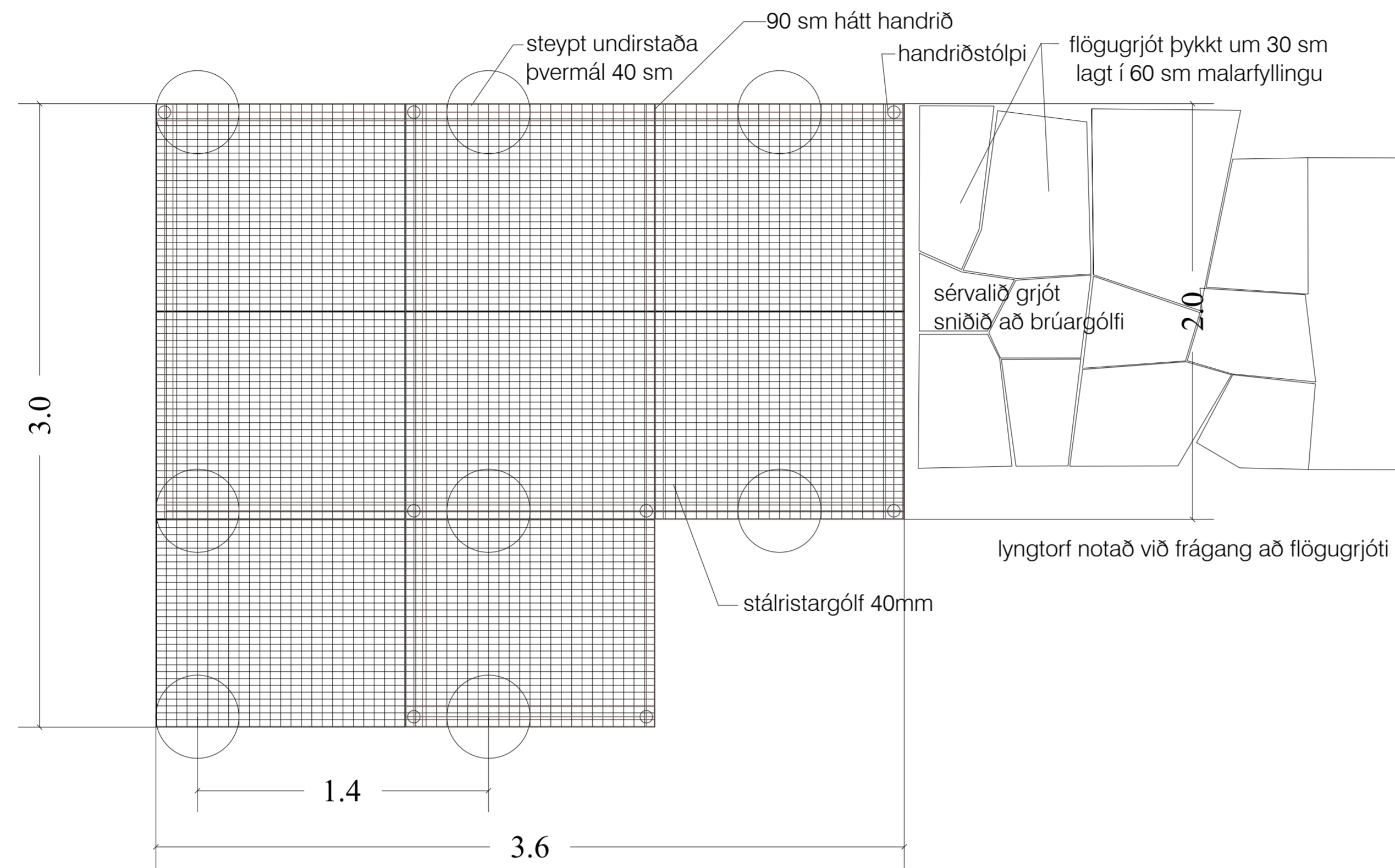
Útsýnispallur III undirbygging mkv: 1. 20
